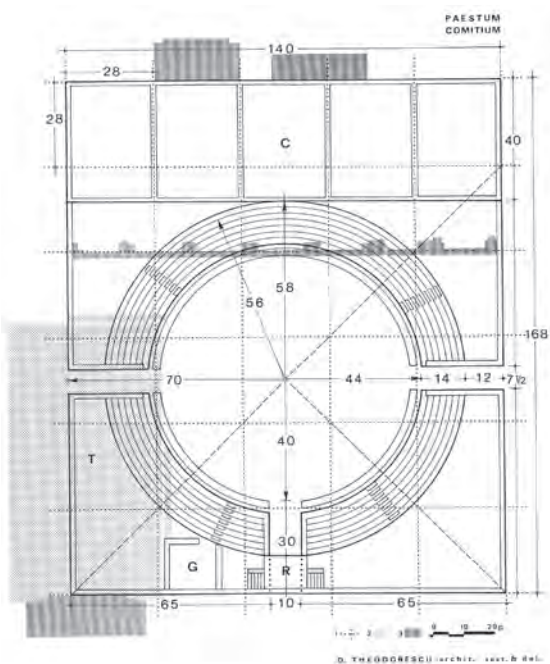
Fig. 13. Plan de l'ensemble comitium-curia à Paestum (D. Theodorescu, Comitium. Le projet , in Poseidonia – Paestum, III, Forum Nord (CEFR 42), E. Greco, D. Theodorescu (éd.), Rome 1987, fig. 41).
