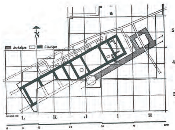
Fig. 3. Kition-Bamboula, le Bâtiment sud (en noir), la muraille (en hachures), le réseau d'égouts et de canalisations (en blanc) (O. Callot, Mission de Kition).
