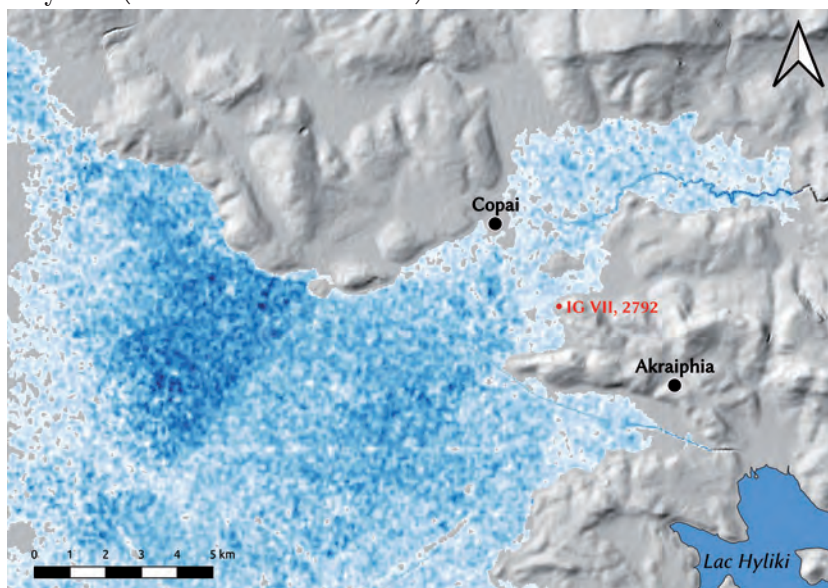
Fig. 9. Simulation de l'étendue du lac dans la baie de Képhalari, hypothèse d'une crue importante (niveau de l'eau = 97 m). © DAO Th. Lucas 2021.
