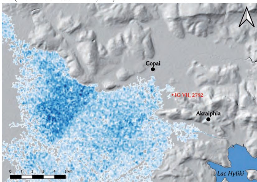
Fig. 7. Simulation de l'étendue du lac dans la baie de Képhalari, hypothèse d'une crue basse (niveau de l'eau = 95,5 m). © DAO Th. Lucas 2021.
