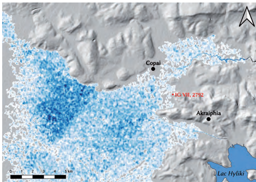
Fig. 8. Simulation de l'étendue du lac dans la baie de Képhalari, hypothèse d'une crue moyenne (niveau de l'eau = 96 m). © DAO Th. Lucas 2021.
