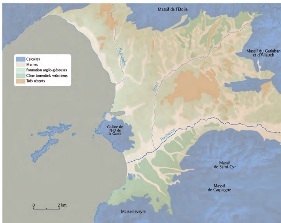
Fig. 2. La situation géomorphologique de la plaine de Marseille (P. Pentsch, Aix-Marseille Université).
