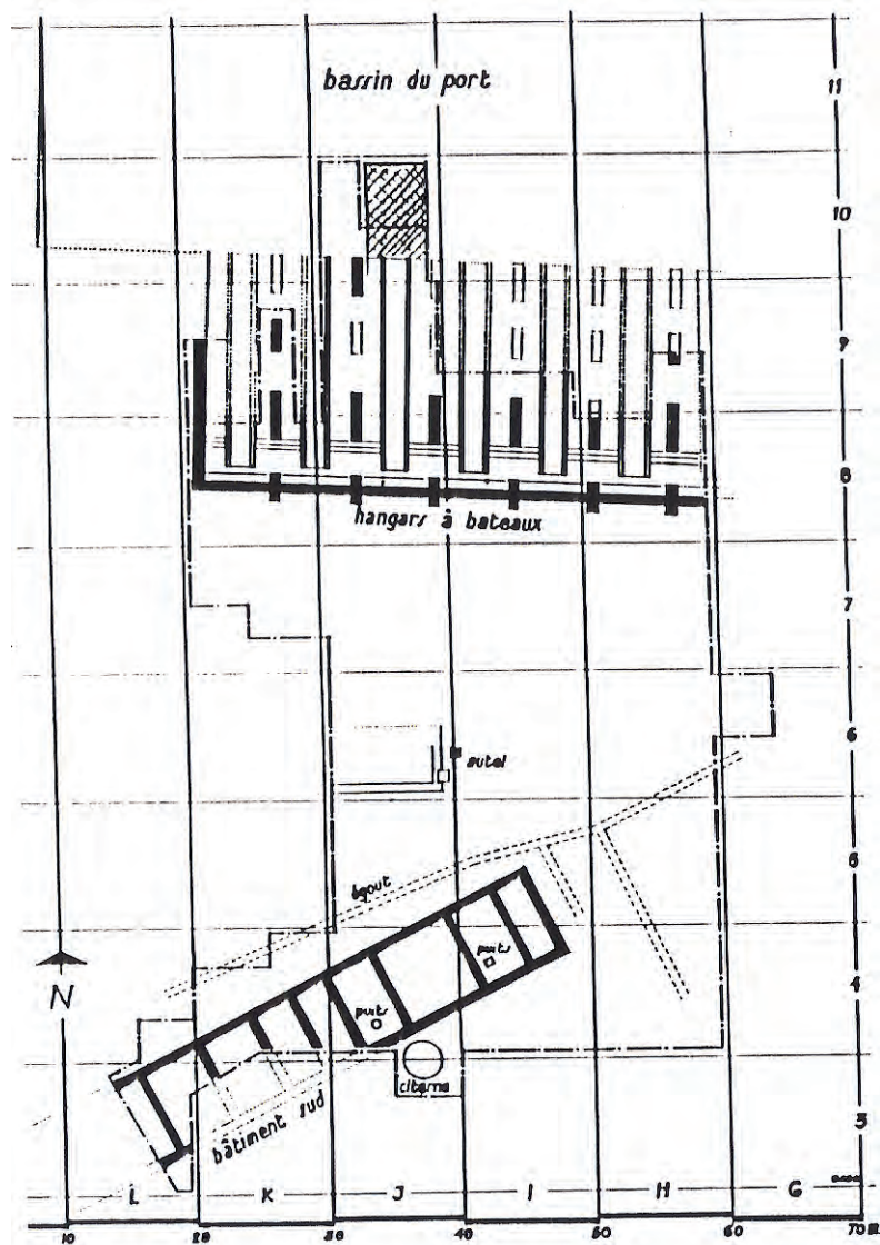
Fig. 7. Plan simplifié des vestiges de Kition-Bamboula en 1987 (O. Callot, Mission de Kition).
